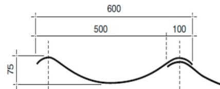
Dimensiones en mm
